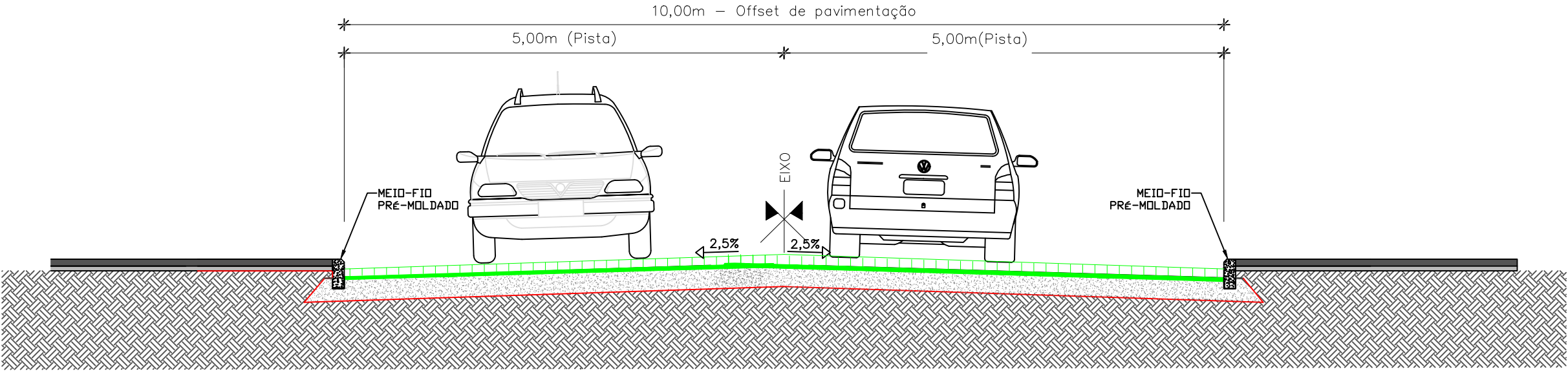
SEÇÃO TIPO DE PAVIMENTAÇÃO- Offset de pavimentação com bloco intertravado - RUA JOÃO PEDRO KOELZER
